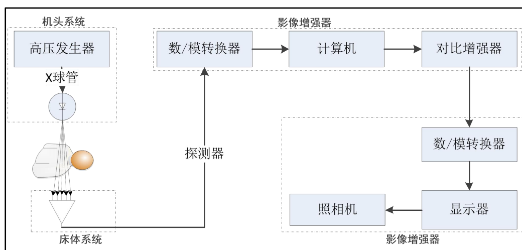
图 9-2 X 射线装置基本原理图
